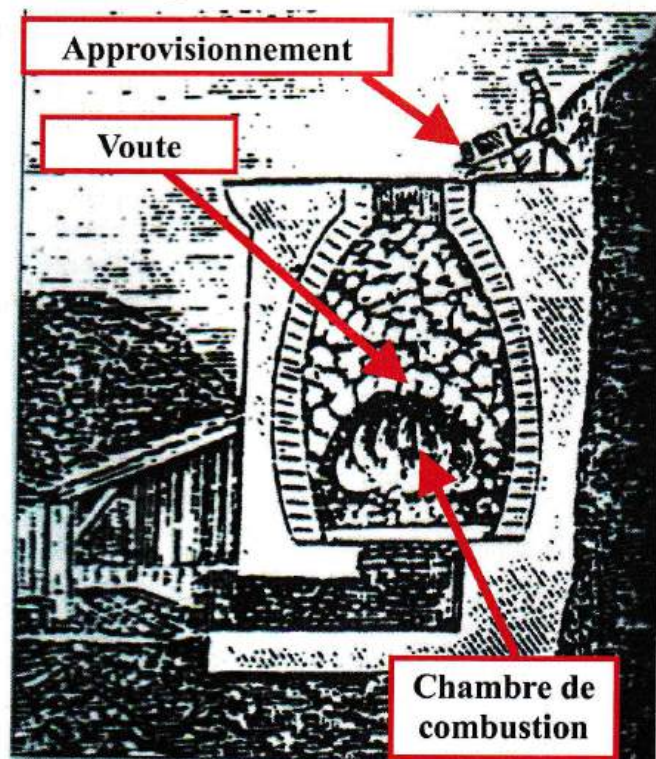
Figure 3 : Vue en coupe d'un four à chaux avec son remplissage par le cratère de la tourelle. Tiré de « L'Agriculture dans les écoles » des frères de l'instruction chrétienne, 1896.
